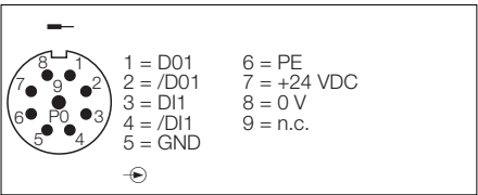
Fieldbus input (M23)
