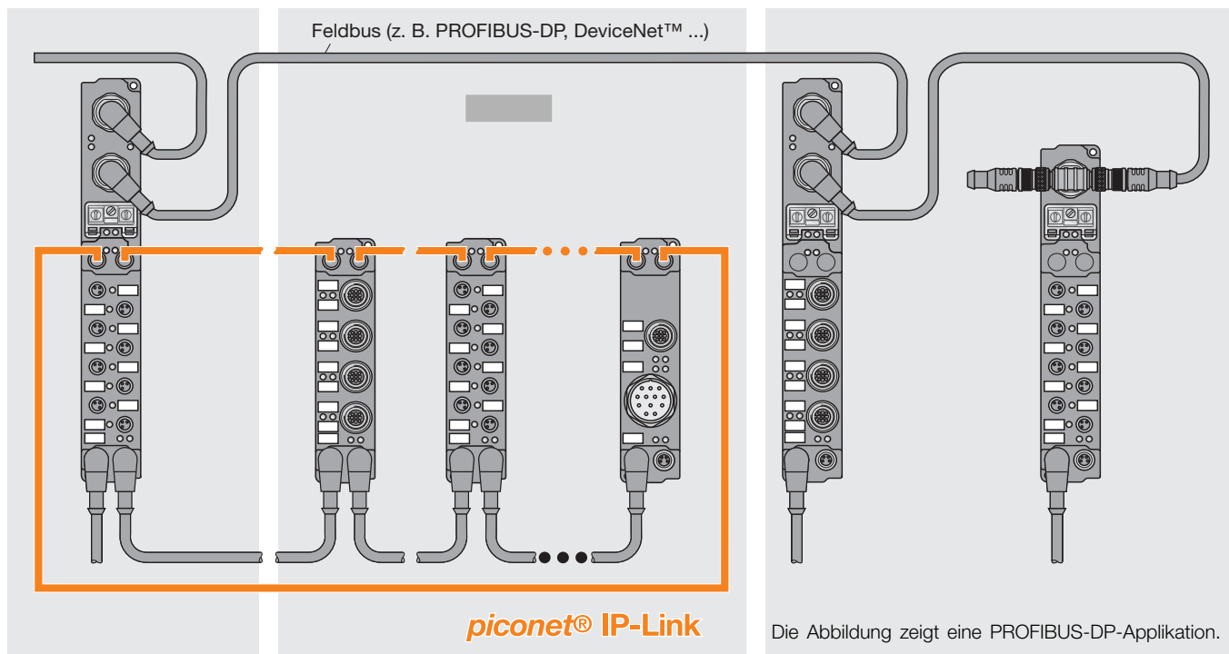
Koppelmodul (Gateway)
